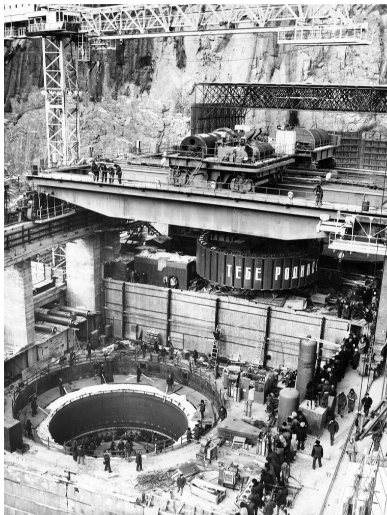
Перенос ротора генератора гидроагрегата № 1 (фото из архива)
