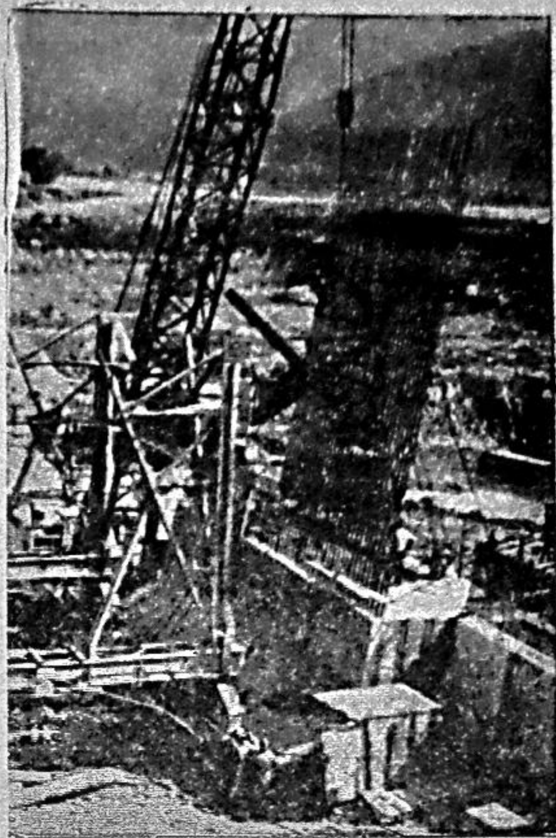
Монтаж крана и армокаркаса левобережной стенки Майнской ГЭС. Фото А. РУДНИЦКОГО.
