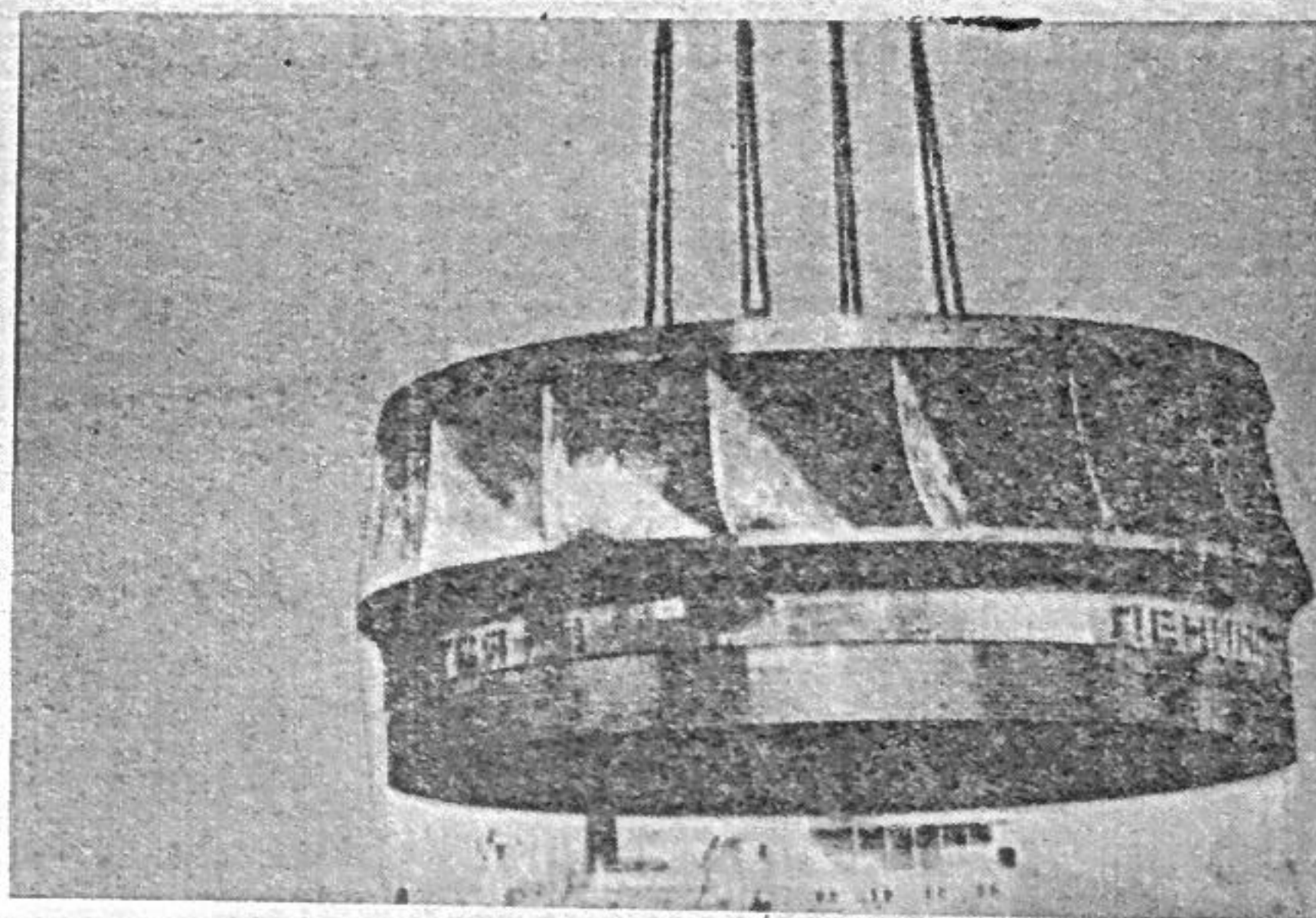
На снимке четвертое рабочее колесо для комсомольского агрегата.
