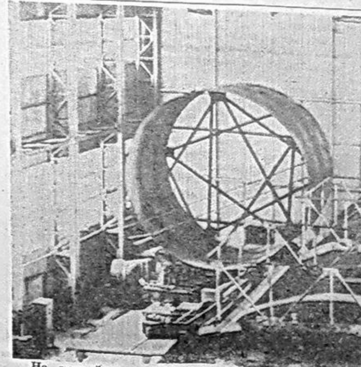
На конвейере кольцо водовода. Фото Н. КАНТА.
