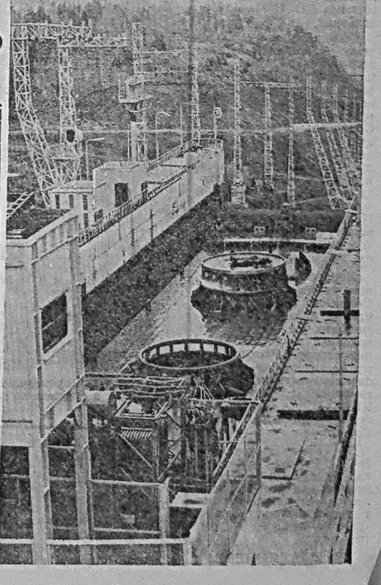
3 октября на строительство Саяно-Шушенской ГЭС доставлено штатное рабочее колесо третьего агрегата. В солнечный яркий день, накануне праздника второй годовщины Конституции СССР, встретили саяногорцы важный груз из Ленинграда. На снимках: штатное рабочее колесо; во время прохождения груза через судовозную камеру судоподъемника Красноярской ГЭС. Фото А. КОНЬКОВА.
