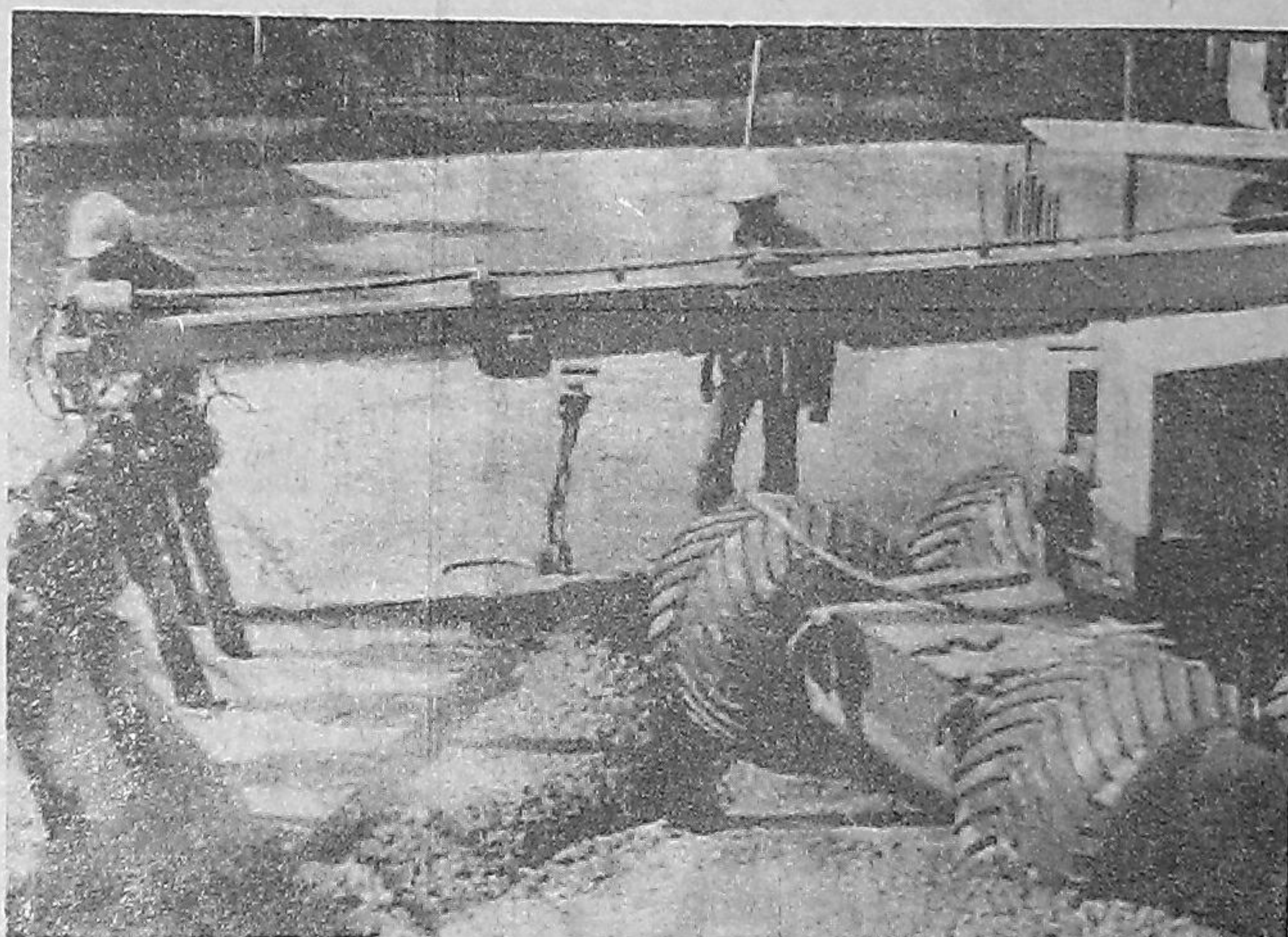
Строительство Саяно-Шушенской ГЭС, укладка бетона при помощи манипулятора.
