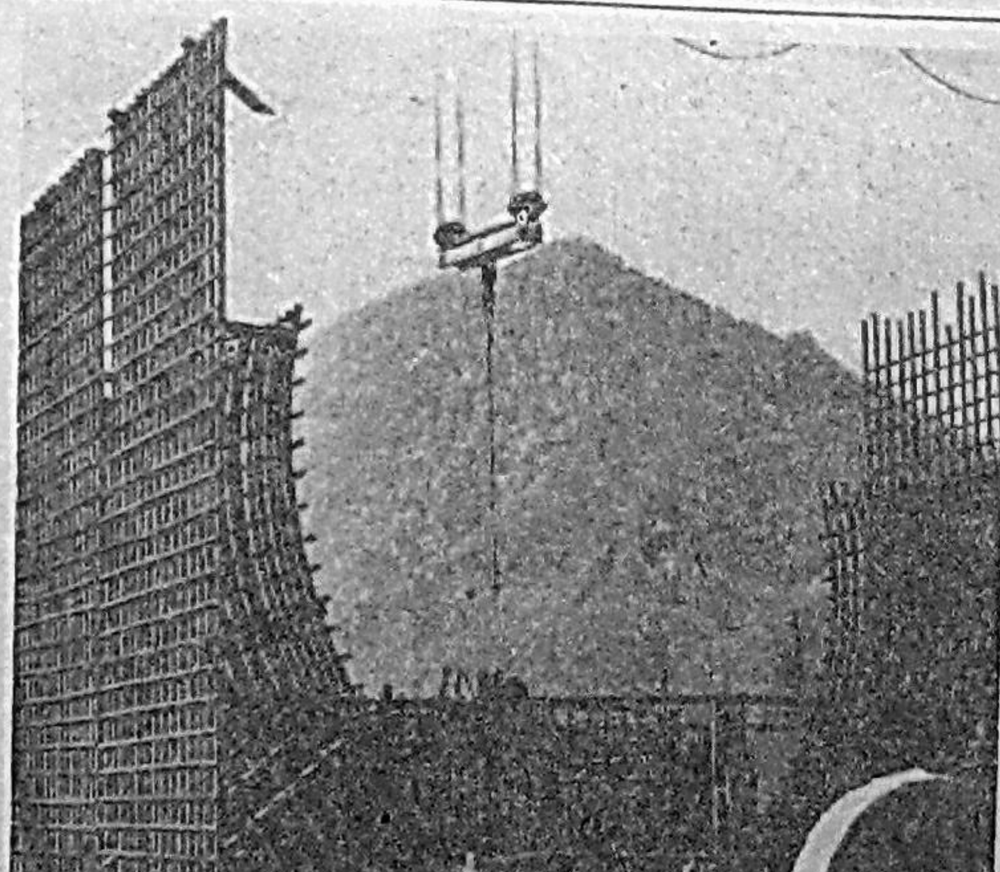
Саяно-Шушенская ГЭС живет большими заботами предпускового этапа второго агрегата. На снимках: из ударных будней стройки.
