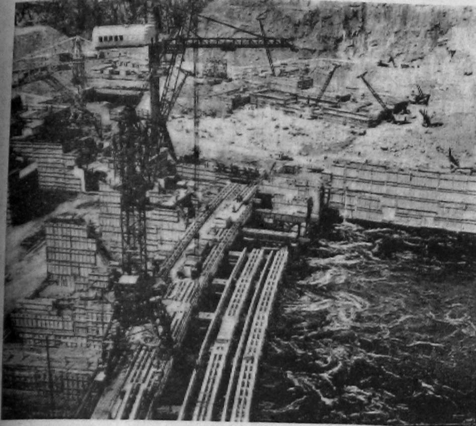
НА СНИМКЕ: главный объект гидростроителей—Саяно-Шушенская ГЭС. В 1973 году она должна дать первый промышленный ток народному хозяйству страны.
