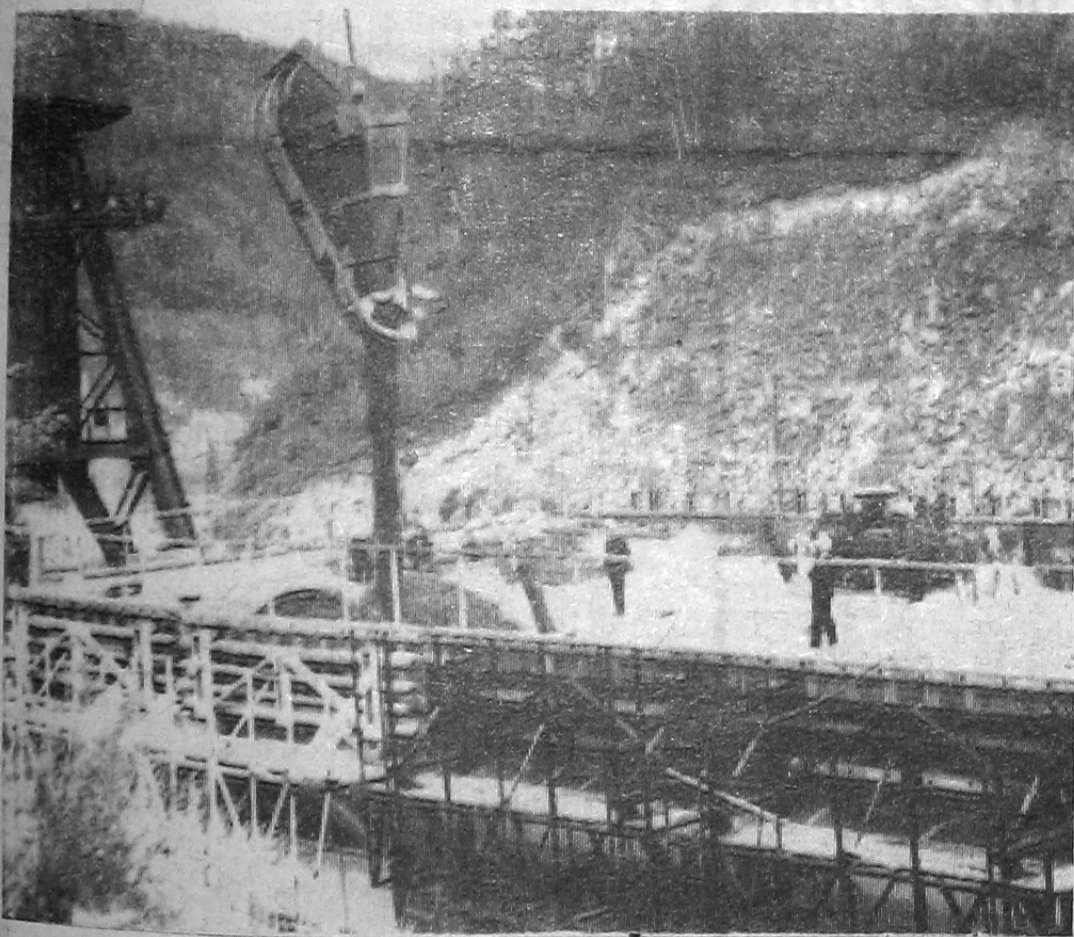
На снимке: идет укладка бетона в блок. Днем и ночью, в выходные дни и в большие торжества плотники-бетонщики, крановщики, автомобилисты несут боевую трудовую вахту на плотине. Каждый гидростроитель стремится сделать как можно больше и лучше, чтобы в 1978 году ГЭС в Саянах дала народному хозяйству первый промышленный ток. Фото Г. КАНУНИКОВА.
