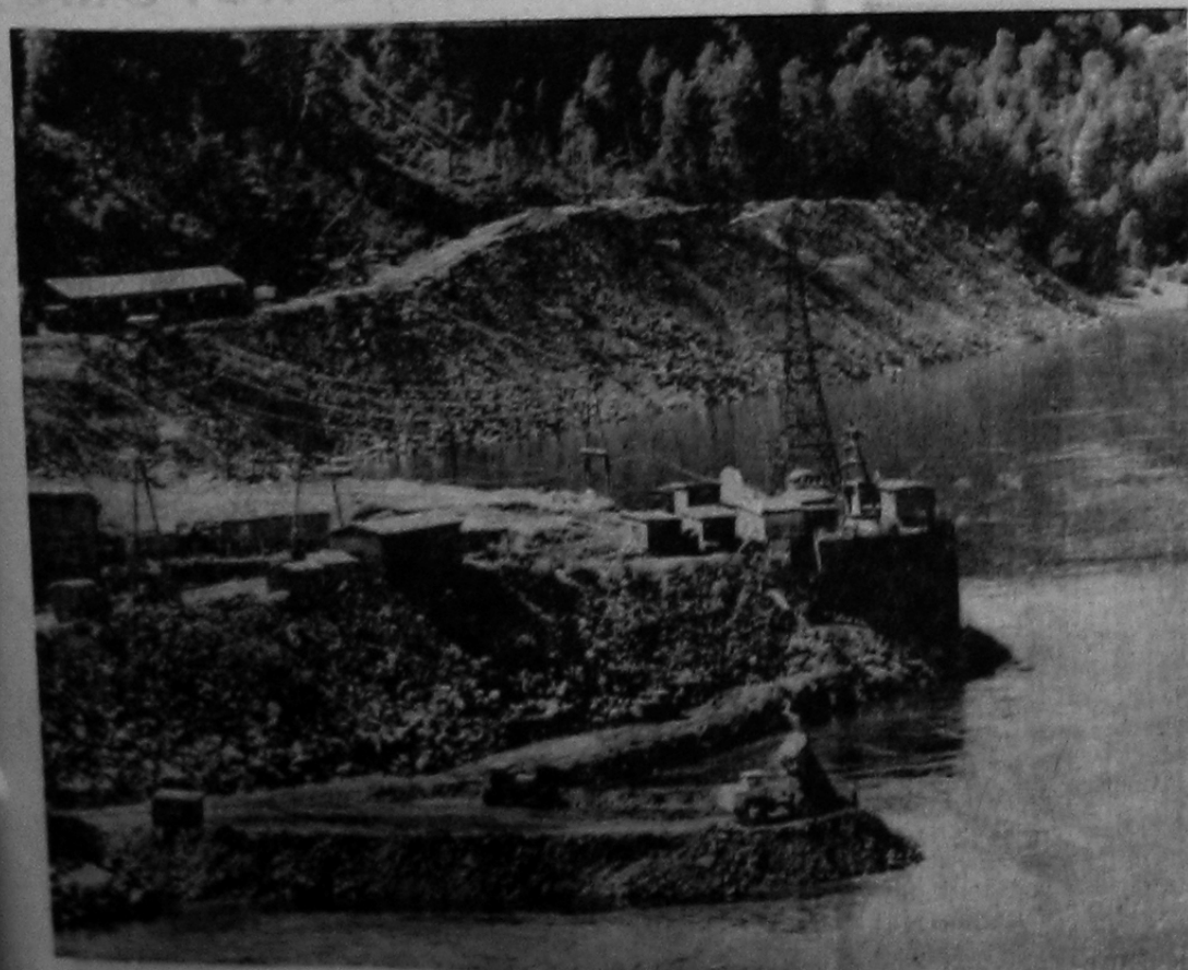
НА ПЕРЕДНЕМ ПЛАНЕ СНИМКА: каменный банкет, который станет перемычкой котлована второй очереди. Отсыпка его началась 31 июля.
