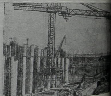
Каждый день вносит изменения в контуры строящейся на Даугаве Рижской ГЭС плотины 50-летия СССР. Основные работы ведутся сейчас там, где сооружаются спиральные камеры, в конусах которых будут монтироваться статоры турбин. Общая мощность — 384 тысячи киловатт.
